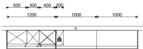
Draufsicht / Bovenanzicht / Vue du dessus / Plan view
