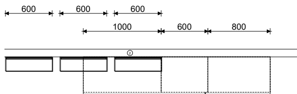
Draufsicht / Bovernaanzicht / Vue du dessus / Plan view
